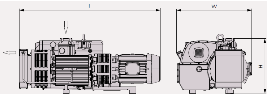
Вакуумний насос RA 0502 C
